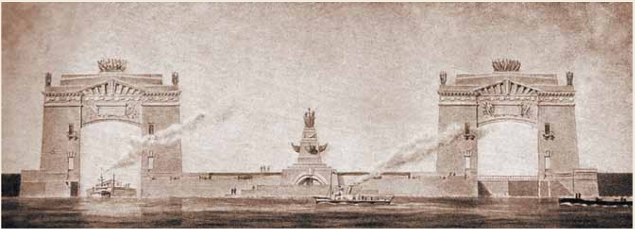
Здание управления верхней головы двухниточного шлюза №14. Вариант проекта. Вид со стороны Цимлянского водохранилища
